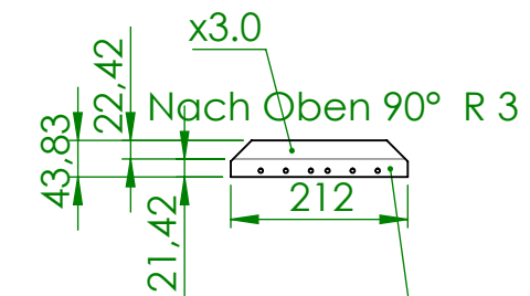
ZC(VUT)x-106 - Profil für Gitter kurz ZCVSM-ROZŁOŻONY-MODEL
