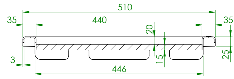
SCHNITT A-A
